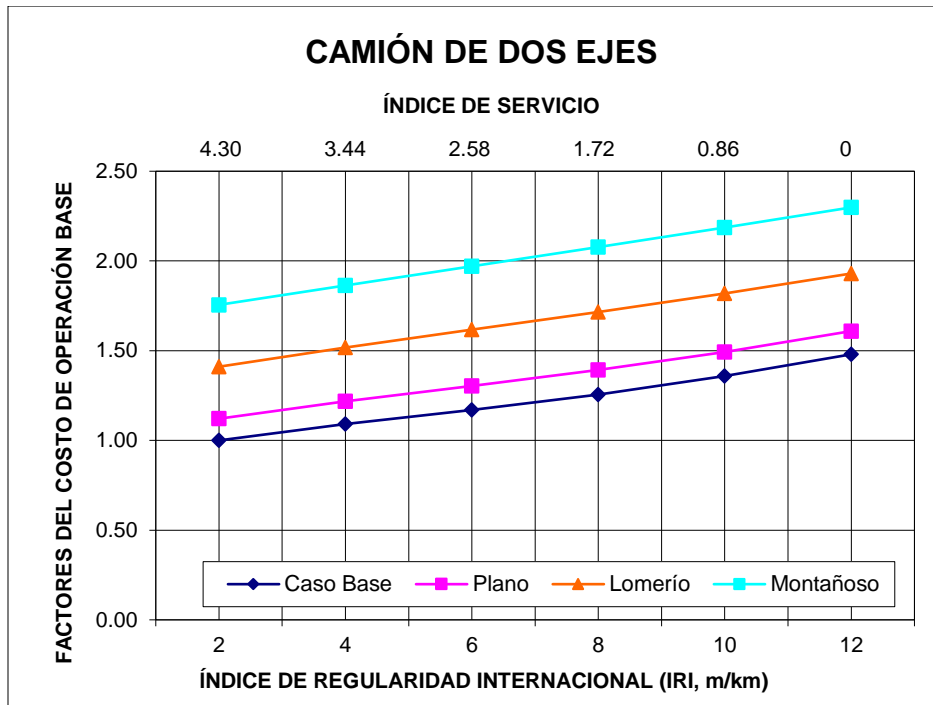
Figura 1.10 Factores del costo de operación para el C2
