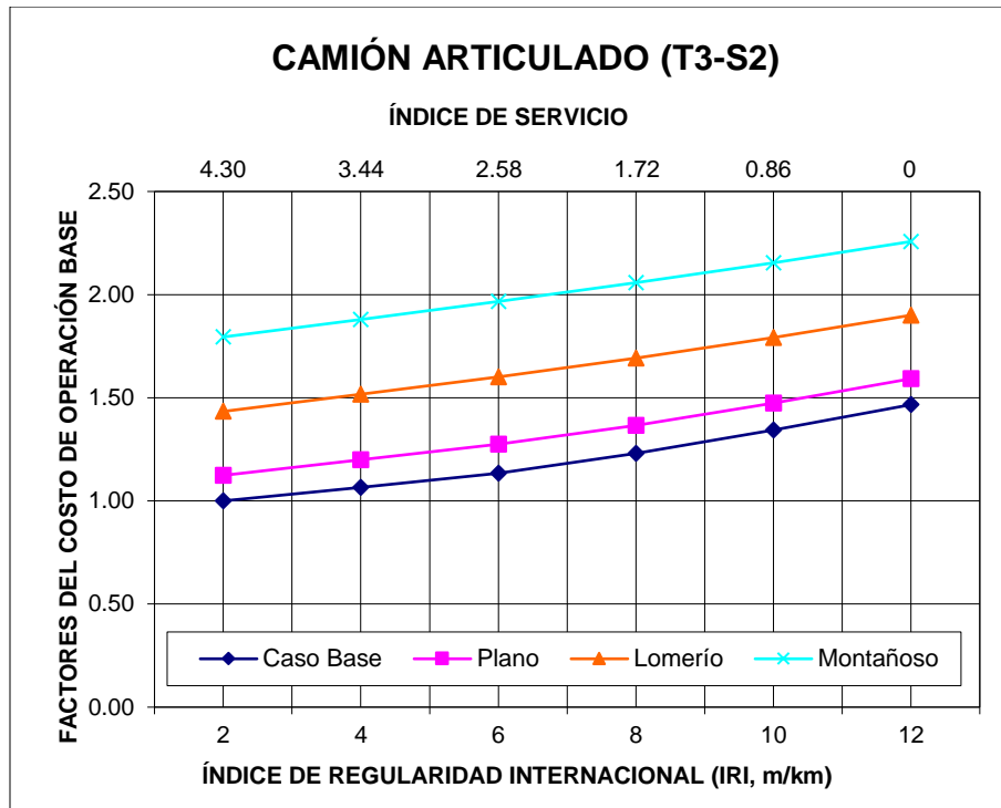
Figura 1.4 Factores del costo de operación para el T3-S2
