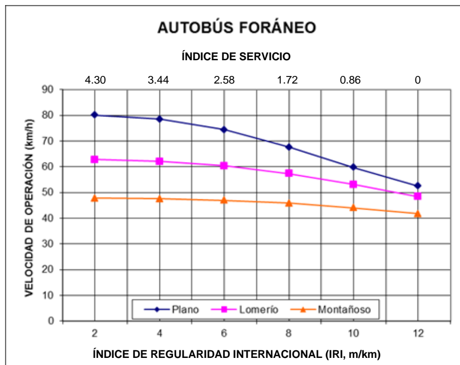
Figura 1.13 Velocidades de operación para el Autobús
