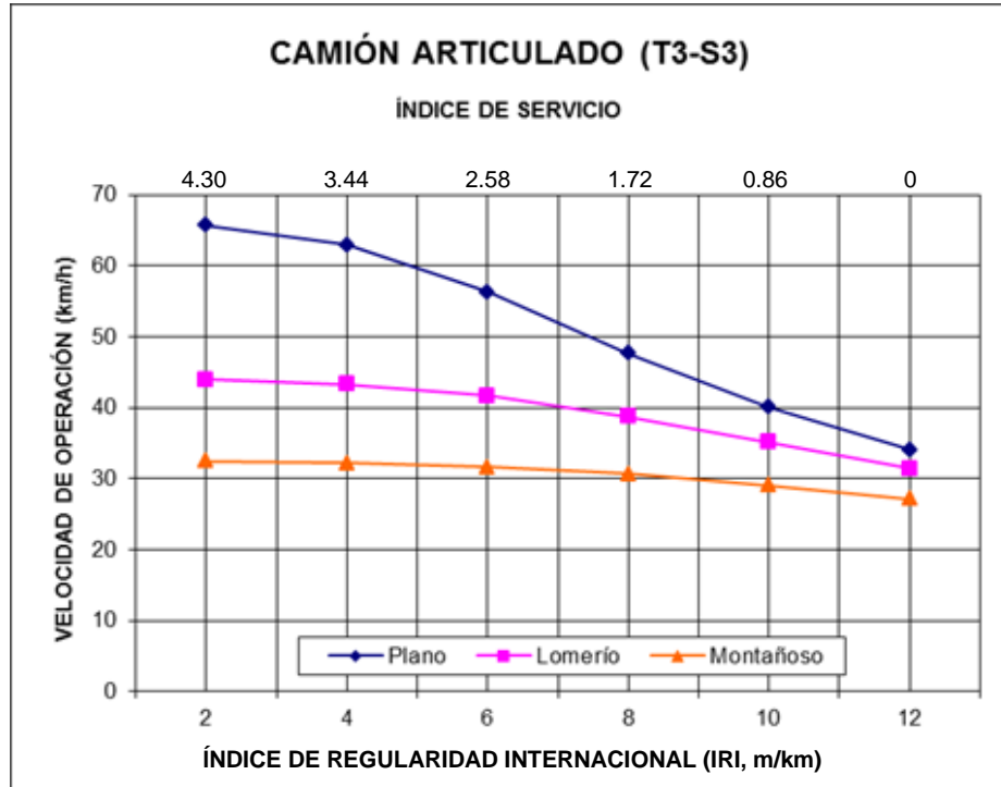
Figura 1.3 Velocidades de operación para el T3-S3
