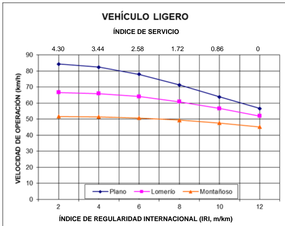
Figura 1.15 Velocidades de operación para el Vehículo Ligero
