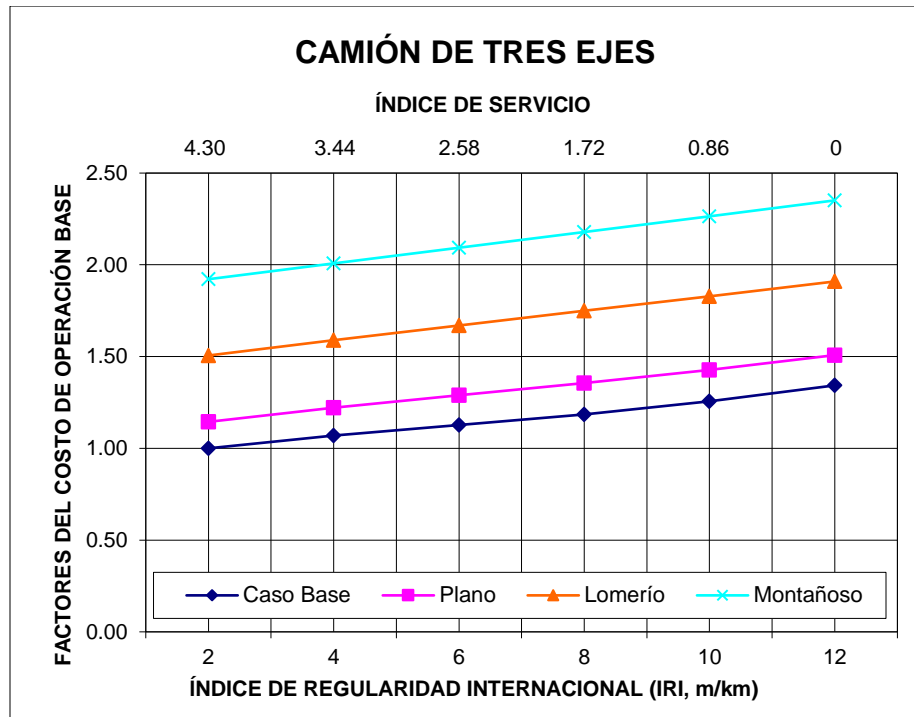
Figura 1.8 Factores del costo de operación para el C3
