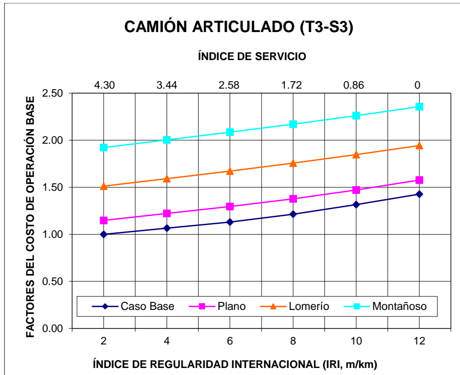
Figura 1.2 Factores del costo de operación para el T3-S3
