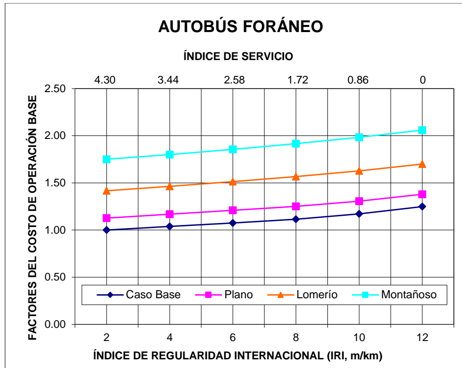
Figura 1.12 Factores del costo de operación para el Autobús
