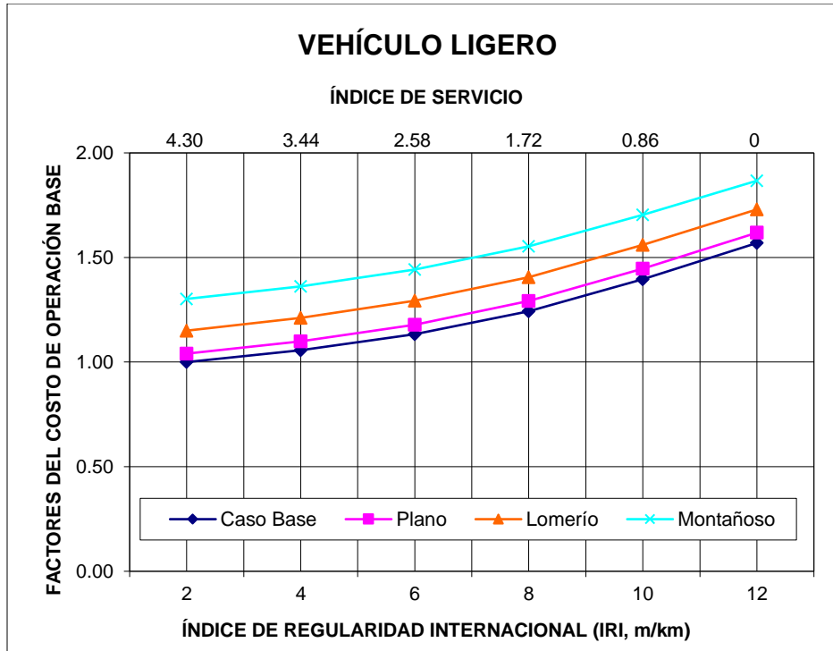
Figura 1.14 Factores del costo de operación para el Vehículo Ligero
