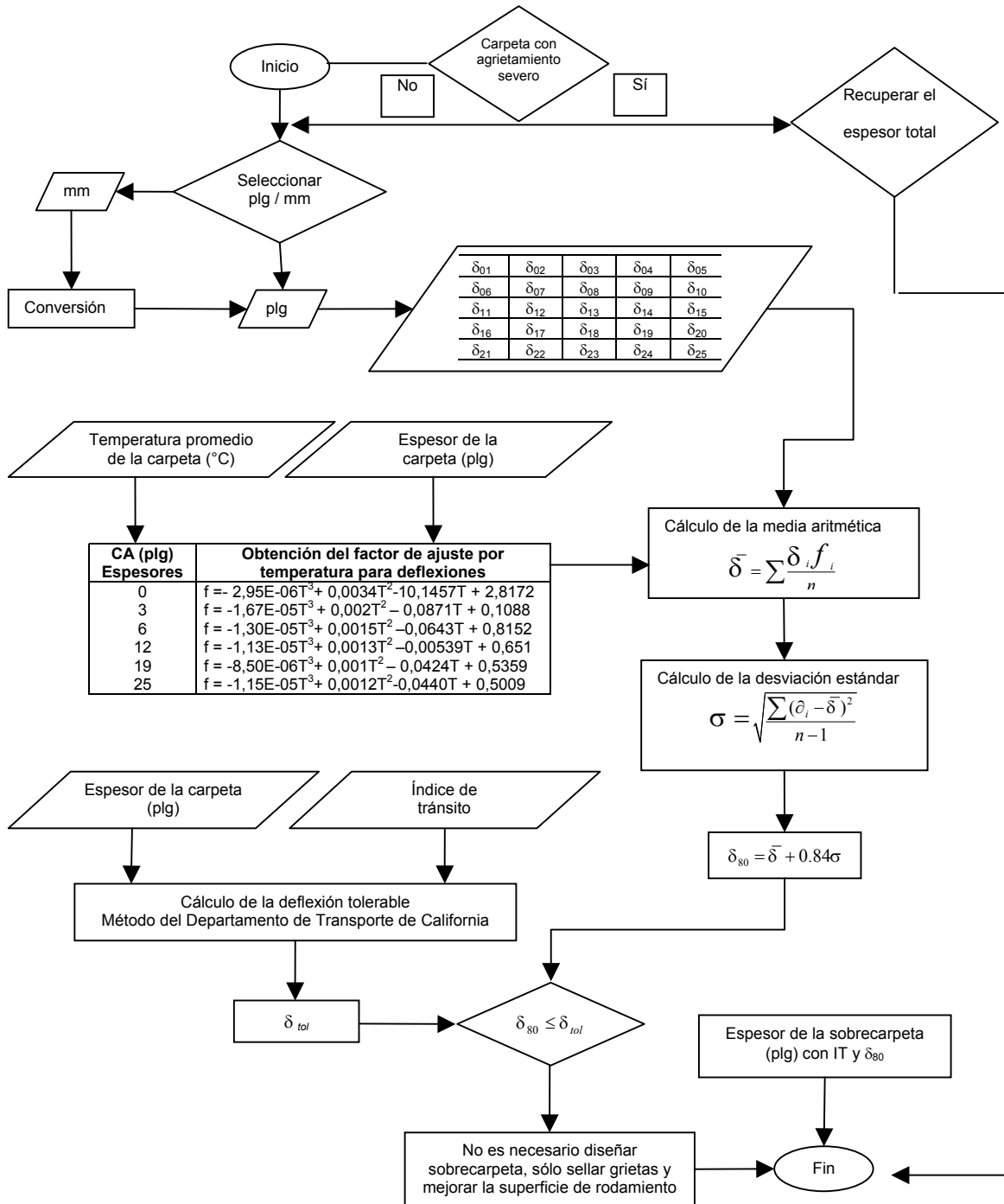
Fig 6.1 Diagrama de flujo para el diseño de sobrecarpetas
