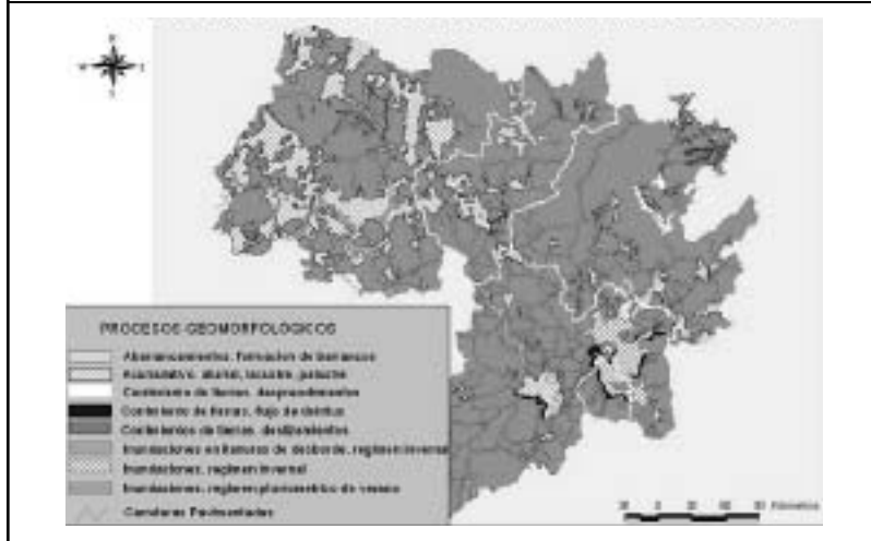
Figura 3.3 Procesos geomorfológicos que afectan la infraestructura carretera en la zona de estudio
