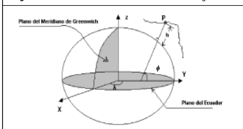
Figura 1.32 Transformación de coordenadas cartesianas en geodésicas
